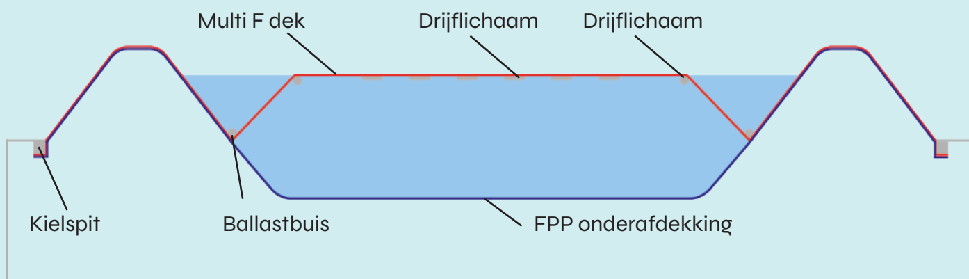
Doorsnede gesloten systeem
