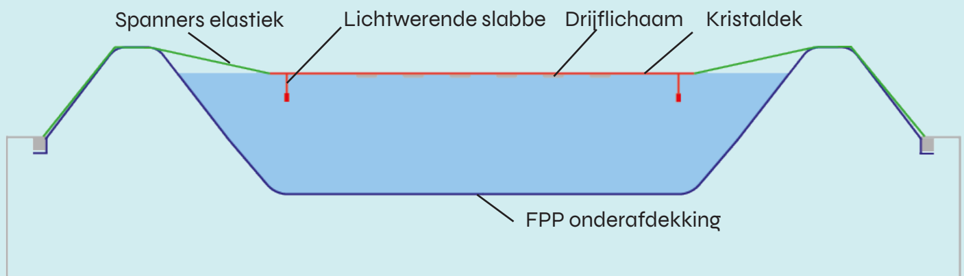
Doorsnede Kristaldek
