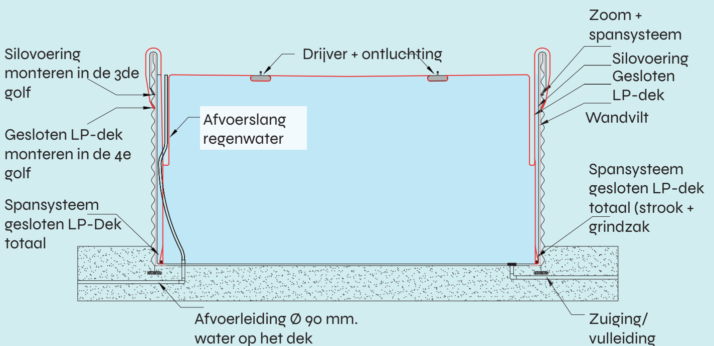
Overzicht gesloten LP-dek
