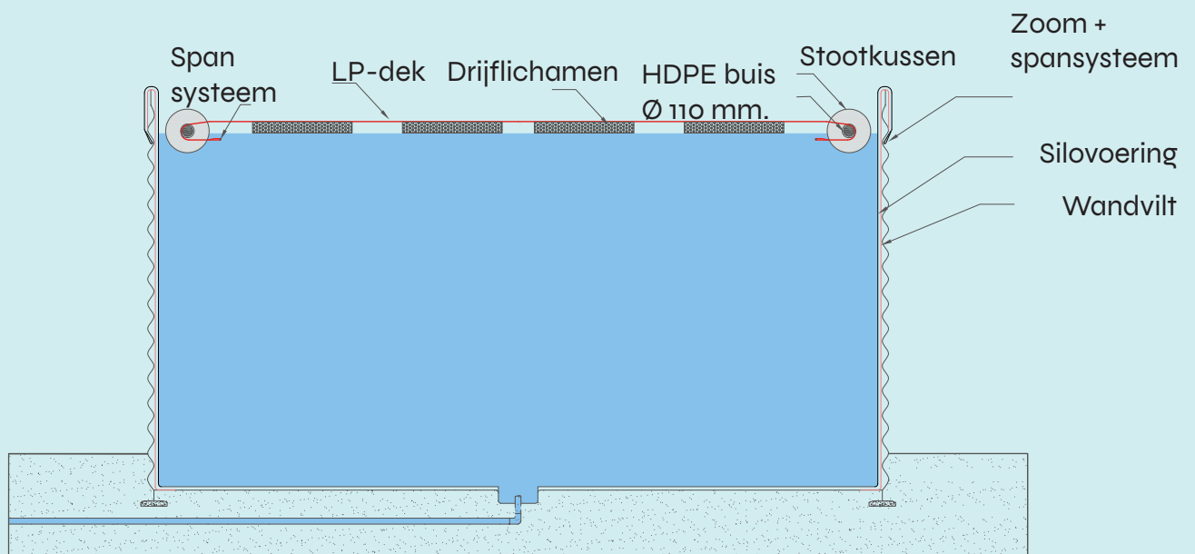
Overzicht LP-dek
